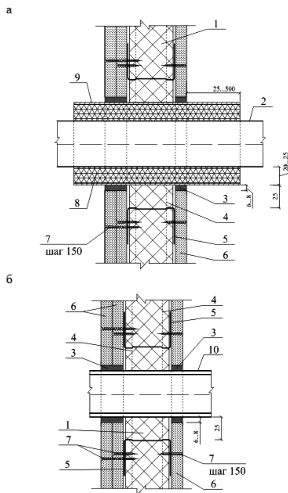
а - при устройстве гильзы; б - при устройстве кожуха
