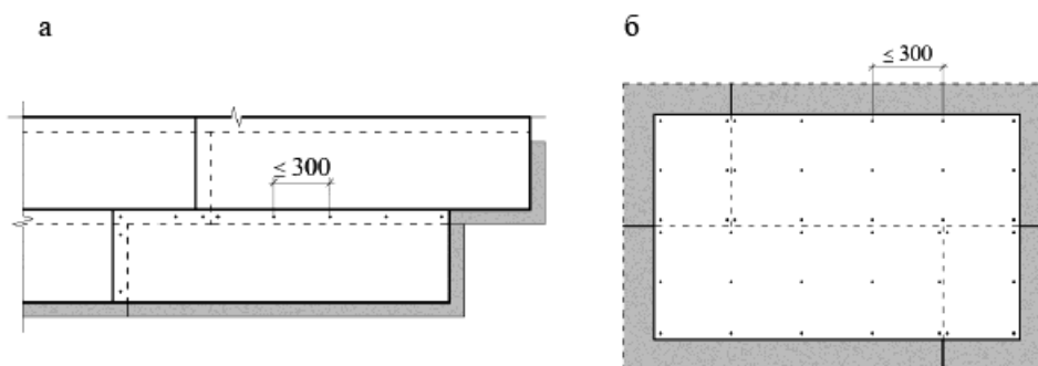
а - крепление ЭП; б - крепление малоформатных ГВЛВ
