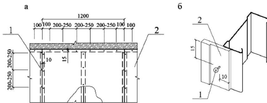
а - общий вид; б - крепление листов к стойке каркаса 1 - самонарезающий винт; 2 - лист ГКЛ или ГВЛ
