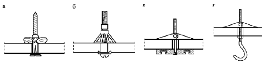
а - дюбель мультифункциональный; б - дюбель для пустотелых конструкций; в и г - анкер проходной
