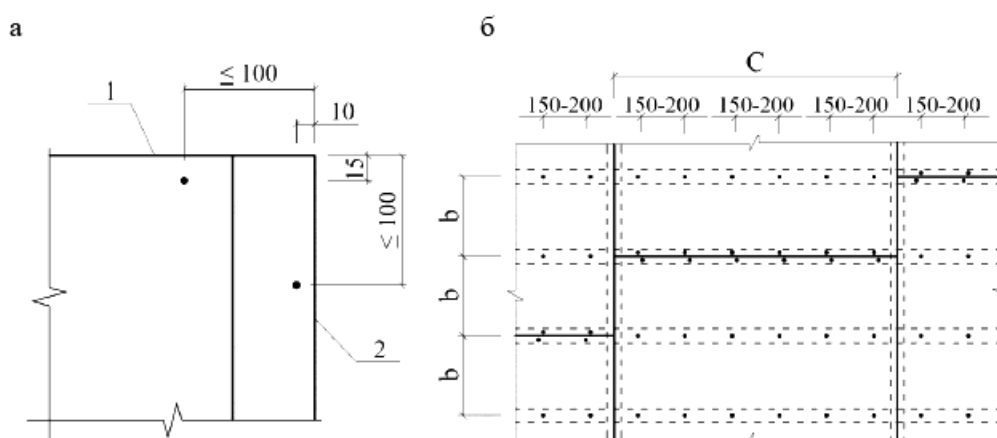
а - схема расположения самонарезающих винтов на краях гипсокартонных листов; б - схема закрепления гипсокартонных или гипсоволокнистых листов к каркасу с помощью самонарезающих винтов 1 - не оклеенная картоном кромка; 2 - оклеенная картоном кромка; C - ширина листа
