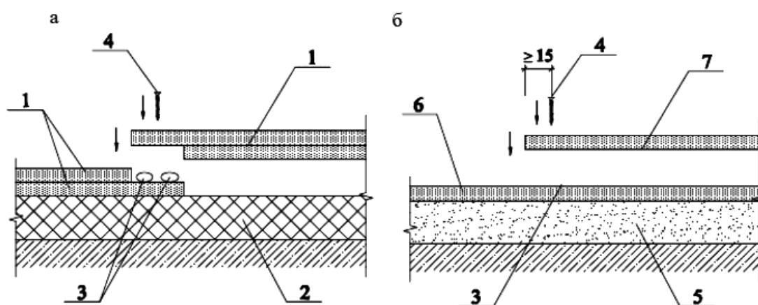
а - соединение ЭП; б - соединение малоформатных ГВЛВ
